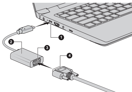
Фигура 4-8 Свързване на RGB кабел към порта за RGB монитор
