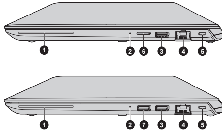
Фигура 3-3 Дясната страна на компютъра
